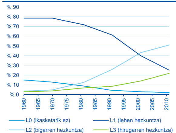
3.1 grafikoa Espainiako 25+ biztanleen frakzioa, hezkuntza-maila bakoitzean
