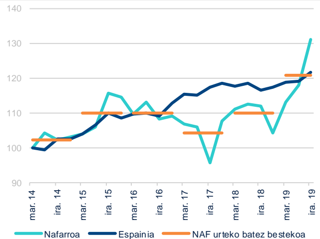
2.17 grafikoa. NAFARROA ETA ESPAINIA: INPORTAZIO ERREALAK (1H14=100, UEEZ)
