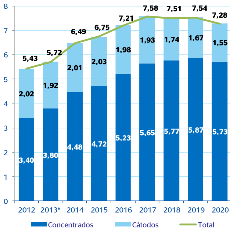
Proyección de producción de cobre (Millones de Toneladas)
